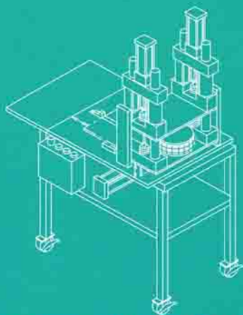
MASSICOT PERFECT BOUND POUR MAGAZINES
