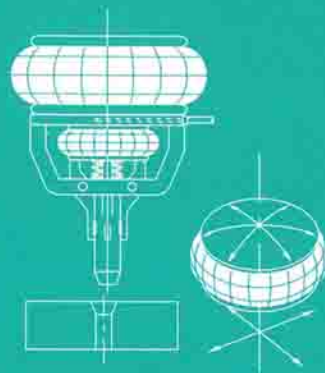
DISPOSITIF D'AUTO-ALIGNEMENT
