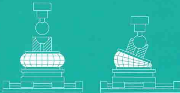
MAINTIEN DE VERTICALITE DE LA VALVE DE CONTROL
