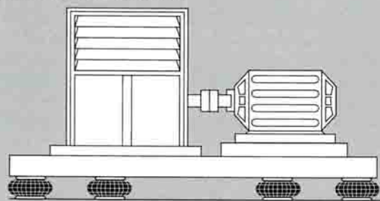
SOUFFLANTE AVEC MOTEUR
