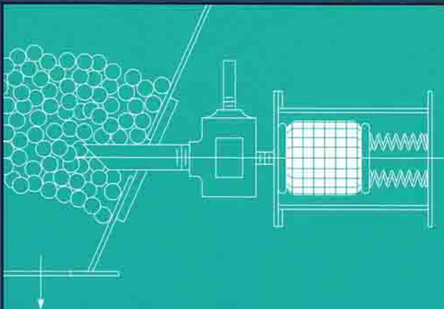
GENERATEUR D'AIR PULSE
